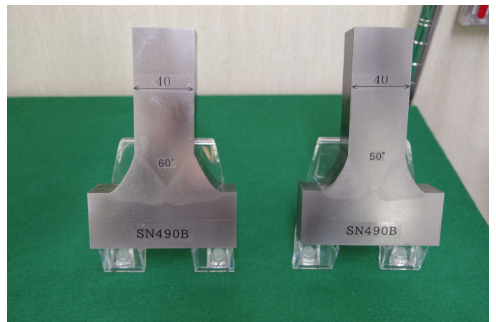
⑫50度開先マクロ試験片
