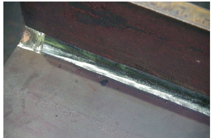
⑩BT材のサブマージ溶接外観
